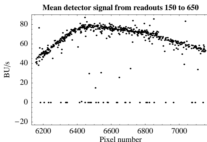
Abbildung 3: Über Orbit 3959 gemitteltes Detektorsignal von Kanal 7, ohne Dead/Bad Pixels.
