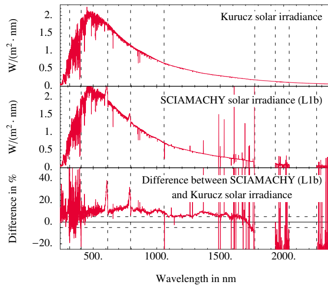
Abbildung 6: Von SCIAMACHY gemessene solare Irradianz SMR_{L1b} im Vergleich mit einem Kurucz Spektrum, Offset von ca. +10 %, Kanäle 7 und 8 von Eisbildung betroffen, SCIAMACHY Kanalgrenzen durch gestrichelte vertikale Linien markiert
