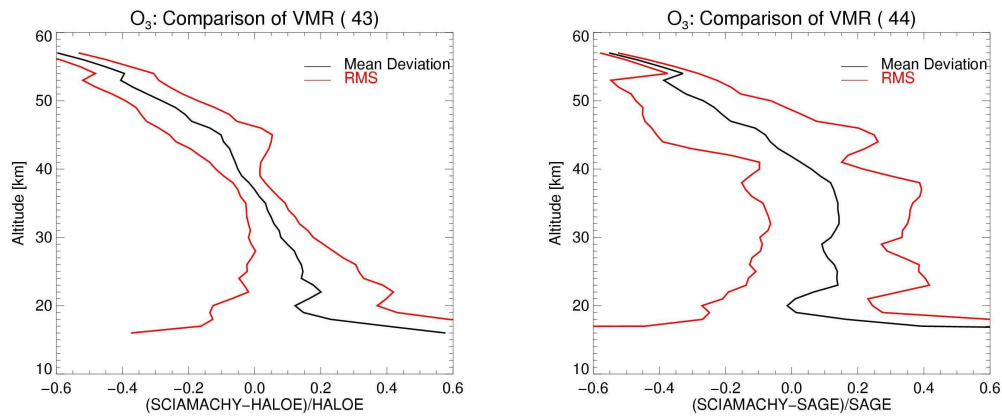
Abbildung 9: Mittlere relative Abweichung (schwarz) und deren Standardabweichung (RMS, rot) aller Kollokationen des Validationsdatensatz von SCIAMACHY-O 3 -Profilen v2.1 zu HALOE v19 (links) und SAGE II v6.2 (rechts). Aus Bracher et al. 2004b
