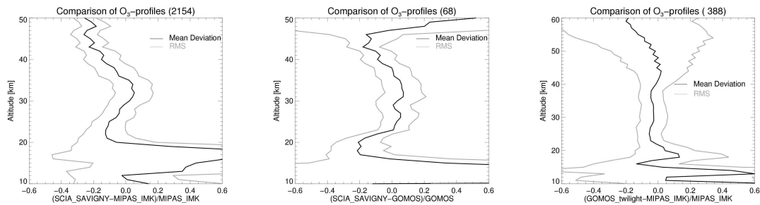
Abbildung 16: Statistische Ergebnisse aller Vergleiche von kollozierten O_3 -Profilen von Okt-Nov 2003 mit mittlerer relativer Abweichung (schwarz) und Standardabweichung der mittleren relativen Abweichung (RMS; grau) bestimmt von allen kollozierten MIPAS_IMK und SCIAMACHY_IUP (SCIA_SAVIGNY; links), SCIAMACHY_IUP und GOMOS (mitte), und MIPAS_IMK und GOMOS (rechts) Messungen. Abb. aus Bracher et al. 2005c
