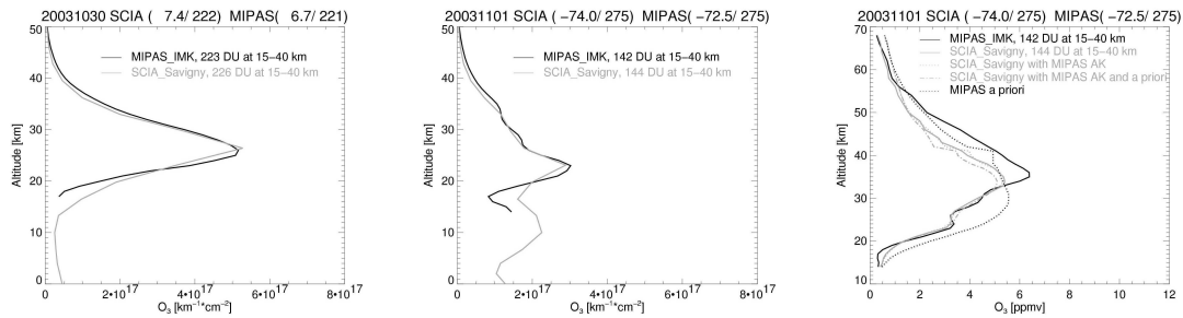
Abbildung 14: Vergleich von O_3 -Profilen kollozierter MIPAS_IMK (schwarz) und SCIAMACHY_IUP (= SCIA_Savigny; grau) Messungen. Beispiele vom 30. Okt und 1. Nov 2003 in den Tropen (links) und hohen südlichen Breiten (mitte) in Teilchendichten und Angabe der Teilsäule von 15 bis 40 km in der Legende. Rechts: Beispiel in den hohen Breiten in VMR von MIPAS_IMK (schwarz, durchgezogen) und SCIA_Savigny (grau, durchgezogen), zusätzlich auch von MIPAS a priori (schwarz, gepunktet), und dem SCIA_SAVIGNY-Profil, welches mit MIPAS a priori (grau, gepunktet) ausgewertet und mit MIPAS Averaging Kernels gefaltet wurde (grau, \cdot-\cdot ). Abb. aus Bracher et al. 2005c
