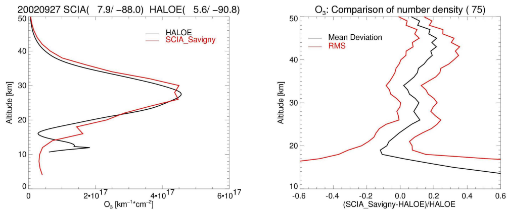
Abbildung 12: Vergleich von Ozonprofilen in Teilchendichten bestimmt aus HALOE-Okkultationsmessungen (schwarz) und aus SCIAMACHY Limbmessungen mit der Retrieval Methode von Savigny et al. 2005 (Version 1.6, rot). Beispiel aus den Tropen (links) und mittlere relative Abweichung (schwarz) und deren Standardabweichung (rot) aller Kollokationen (insgesamt 75). Aus Rozanov et al. 2003
