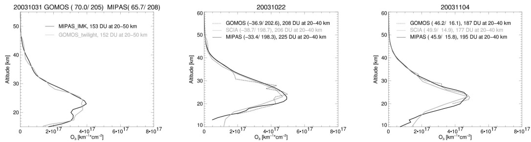
Abbildung 15: Vergleich von O_3 -Profilen kollozierter MIPAS_IMK (schwarz) und GOMOS (grau) Messungen in der Arktis (links) und von Dreier-Kollokationen von MIPAS_IMK (schwarz), SCIAMACHY_IUP (= SCIA; grau) und GOMOS (schwarz, gepunktet) in den nördlichen polaren Breiten (links), Subtropen (mitte) und in den nördlichen mittleren Breiten (rechts). Angabe der Teilsäule von 20 bis 50, bzw. 20 bis 40 km in der Legende. Abb. aus Bracher et al. 2005c
