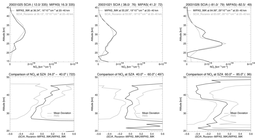
Abbildung 17: Vergleich von \text{NO}_2 -Profilen kollozierter MIPAS_IMK (schwarz) und SCIAMACHY_IUP (=SCIA_Rozanov; grau) Messungen von Okt-Nov 2003. Oben: Beispiele bei verschiedenen Sonnenzenithwinkeln (SZA: \tilde{3}6^\circ (links), \tilde{5}4^\circ (mitte), \tilde{8}4^\circ (rechts)), ebenso Angabe der Teilsäule von 20 bis 40 km in der Legende. Unten: Statistische Ergebnisse aller Vergleiche von kollozierten \text{O}_3 -Profilen mit mittlerer relativer Abweichung (schwarz) und Standardabweichung der mittleren relativen Abweichung (RMS; grau) bei verschiedenen SZA-Bereichen: 60^\circ bis 85^\circ (links), 40^\circ bis 60^\circ (mitte), und 24^\circ bis 40^\circ (rechts).
