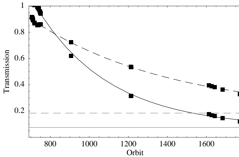
Abbildung 2: Transmission der Eisschicht auf den Kanälen 7 (durchgezogen) und 8 (gestrichelt) aufgetragen vom SRC-Release bis zur Dekontamination ab Orbit 1780
