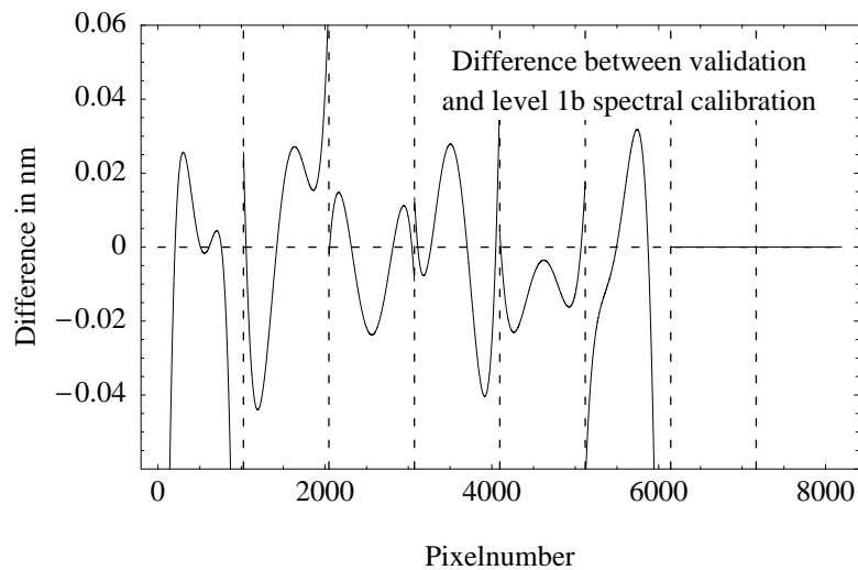
Abbildung 5: Unterschied der mit eigenen Routinen anhand von SLS Messungen im Orbit bestimmten spektralen Kalibration zu der im Level 1b Produkt enthaltenen (Kanalgrenzen sind durch gestrichelte vertikale Linien markiert).
