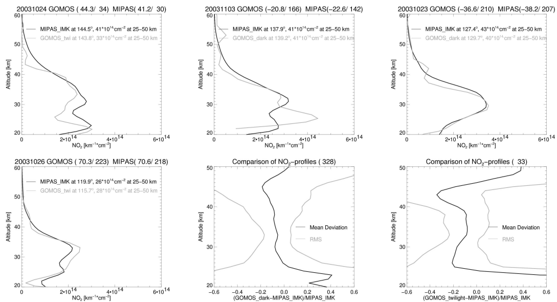
Abbildung 18: Vergleich von \text{NO}_2 -Profilen kollozierter MIPAS_IMK (schwarz) und GOMOS (grau) Messungen von Okt-Nov 2003. Beispiele bei verschiedenen Sonnenzenithwinkeln (SZ: \sim 145^\circ mit GOMOS Dämmerungsmessung (oben links), \sim 138^\circ mit GOMOS Dunkelmessung (oben mitte), \sim 128^\circ mit GOMOS Dunkelmessung (oben rechts), \sim 118^\circ mit GOMOS Dämmerungsmessung (unten links), ebenso Angabe der Teilsäule von 25 bis 50 km in der Legende. Unten: Statistische Ergebnisse aller Vergleiche von kollozierten \text{O}_3 -Profilen mit mittlerer relativer Abweichung (schwarz) und Standardabweichung der mittleren relativen Abweichung (RMS; grau) für alle MIPAS-GOMOS_Dunkel- (unten mitte) und MIPAS-GOMOS_Dämmerungskoinzidenzen (unten rechts).
