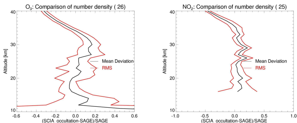
Abbildung 11: Mittlere relative Abweichung (schwarz) und deren Standardabweichung (rot) von Ozonprofilen (links) und NO 2 -Profilen (rechts) bestimmt aus SCIAMACHY-Okkultationsmessungen mit der Retrieval-Methode von J. Meyer et al. (2005) mit SAGE II. Diese statistische Analyse schließt alle koinzidenten Messungen (insgesamt 26) mit ein, die für die vorhandenen SCIAMACHY Level-1-Daten vom 1.7.2003 bis 28.02.2003 mit SAGE II gefunden wurden. Aus Meyer et al. 2005
