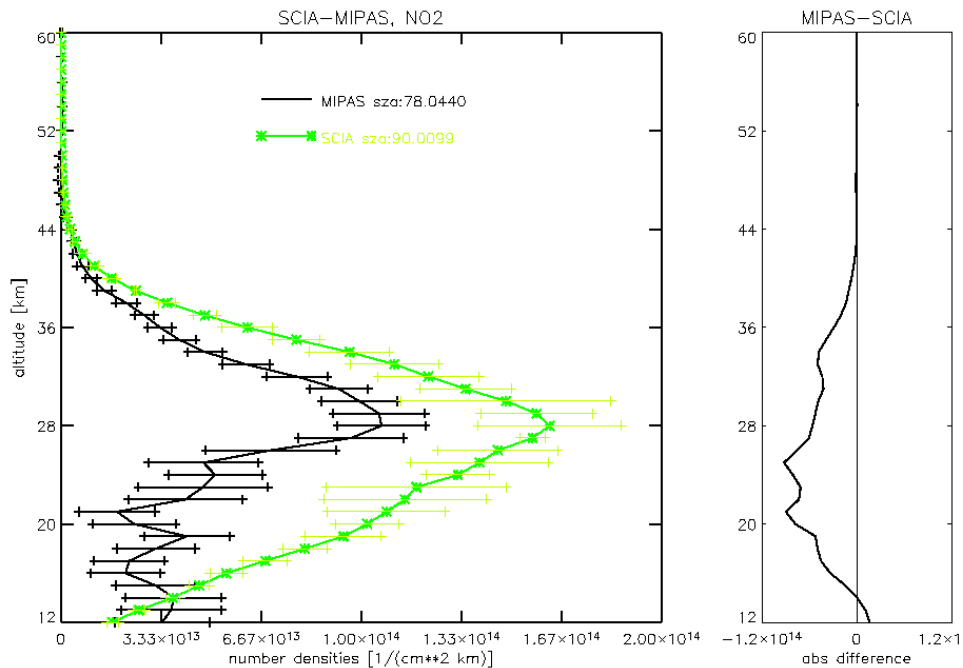
Abbildung 20: Vergleich von MIPAS und SCIAMACHY NO 2 -Profilen einer geeigneten Kollokation. Die MIPAS Messung erfolgte bei 65,3° N und 48,4° O um 07:01:50 UTC, die SCIAMACHY Messung erfolgte bei 68,1° N und 38,9° O um 13:23:13 UTC. Die Messungen liegen 520 km und 6 h 21 min auseinander. Rechts ist die Differenz der Profile in Teilchenzahldichten dargestellt.
