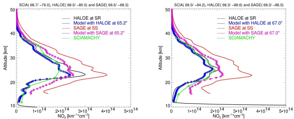
Abbildung 13: Vergleich von mit der Methode von Rozanov et al. (2004) aus SCIAMACHY Level-0-Daten bestimmten NO_2 -Profilen (grün) unterschiedlicher Sonnenzenithwinkel (SZW) mit HALOE NO_2 -Profilen (schwarz) und SAGE II (rot), die bei 90° SZW gemessen wurden und nach Bracher et al. (2004b) auf den SCIAMACHY SZW konvertiert wurden (blau für HALOE und pink für SAGE II). SZW von SCIAMACHY ca. 65° (links), 67° (rechts). Aus Bracher et al. (2005a)
